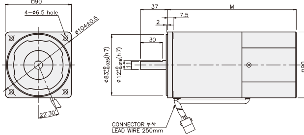
치수도표
